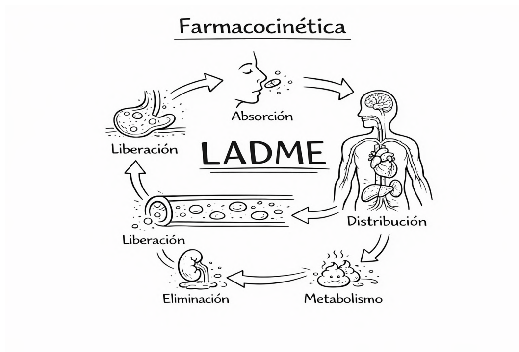
Figura 9.2: Farmacocinética (LADME)
