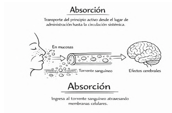
Figura 9.4: Absorción
