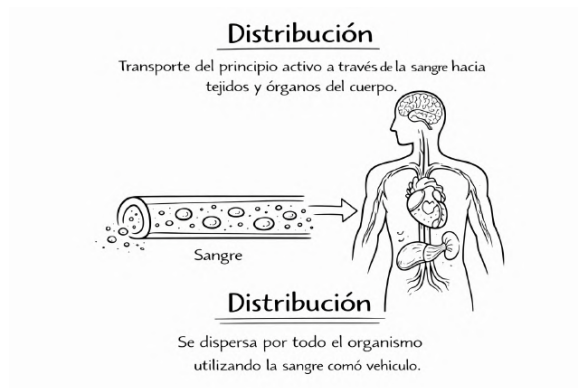
Figura 9.5: Distribución
